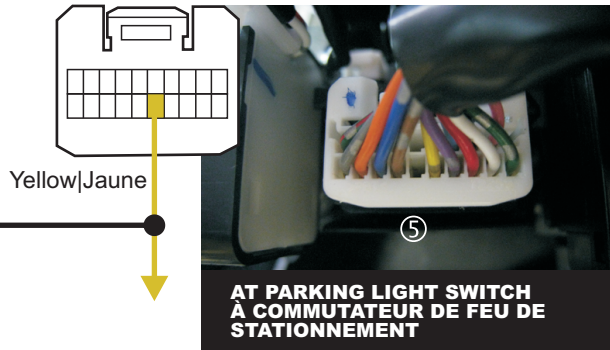
⑤ BACK VIEW VUE DE DOS
